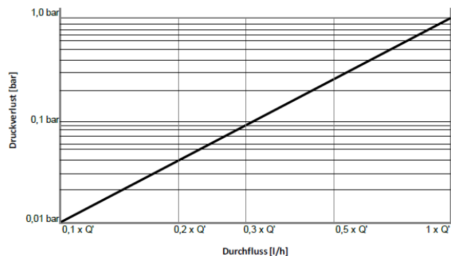
Typische Druckverlustkurve
